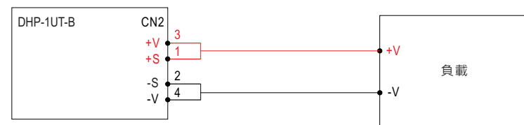
圖5-9 Local Sense配線示意圖
