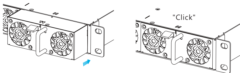
圖3-2 NCP-3200置入機箱示意圖
