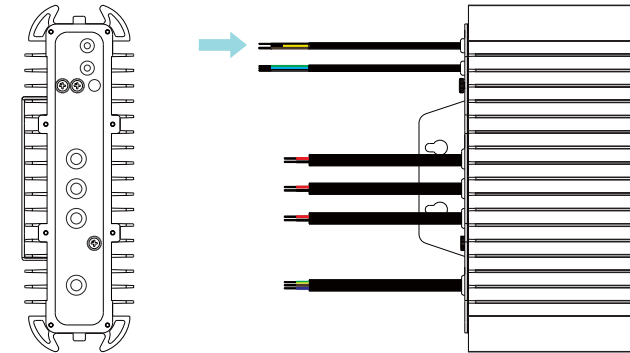
UL2517 22AWG×3C
